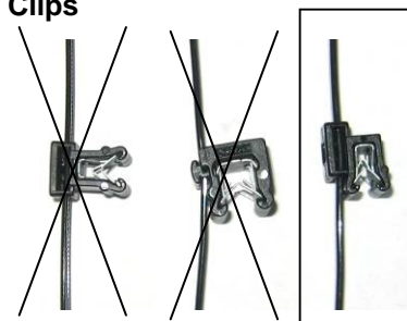
Edge Clips
