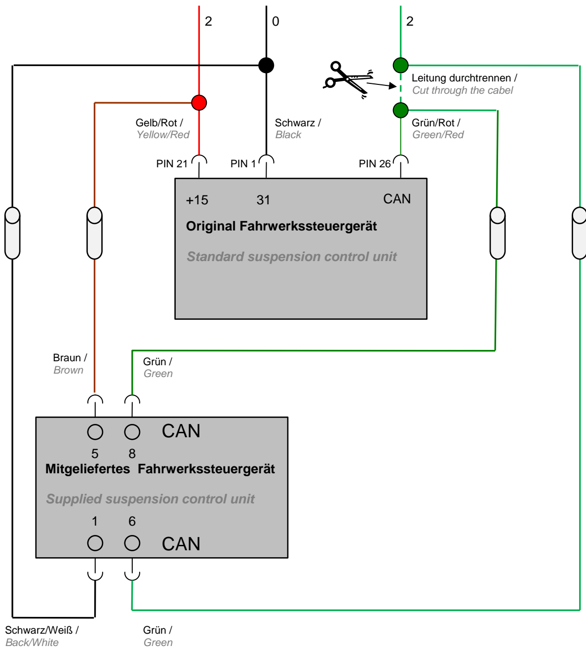
Schaltplan 1 Fahrwerkssteuerg rät / Connection diagram 1 suspension control unit
